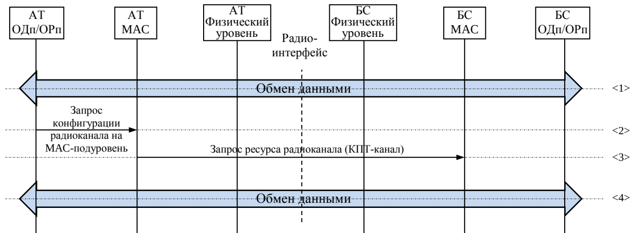
Рисунок 52 – Процедура «Периодический отчет АТ об используемой ширине полосы радиоканала»
