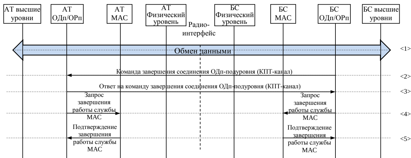
Рисунок 57 – Процедура «Завершение соединения ОДп-подуровня по инициативе БС»
