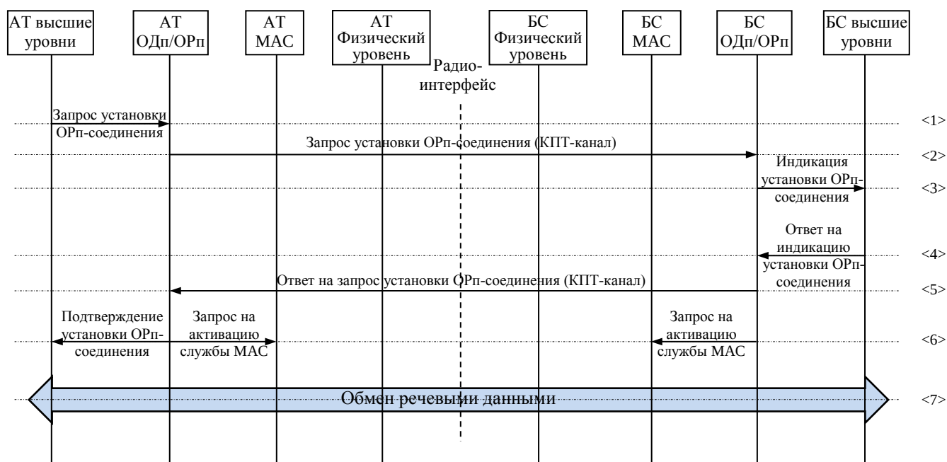
Рисунок 45 – Процедура «Установка соединения ОРп-подуровня по инициативе АТ» при наличии соединения с МАС-подуровнем БС
