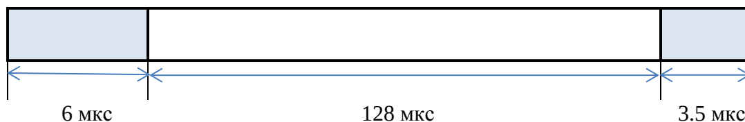
Рисунок 8 – Временная структура OFDMA-символа
