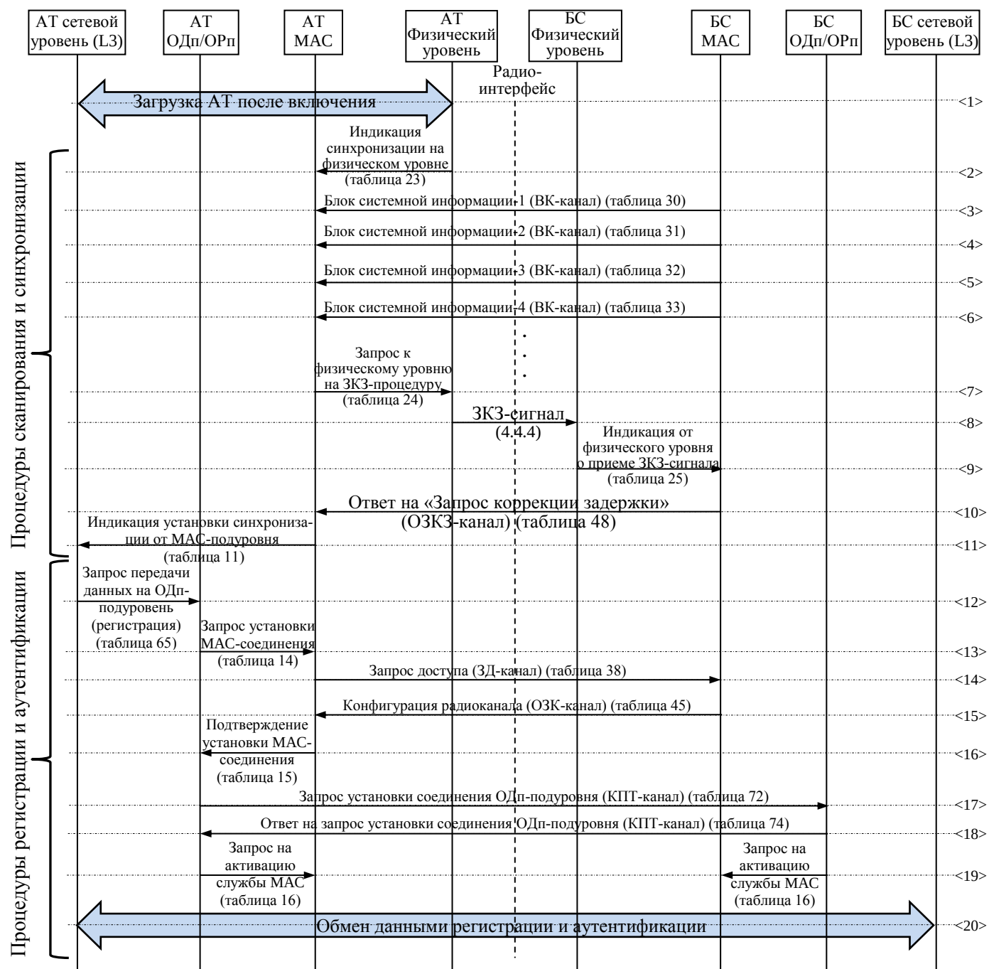
Рисунок 62 – Процедура «Доступ к сети и инициализация»
