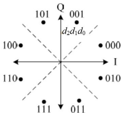
Рисунок 5 – Созвездие 8PSK
