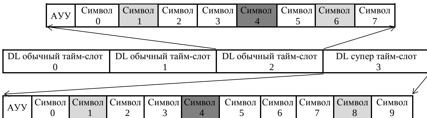
Рисунок 14– Структура тайм-слотов в кадре трафика в DL длительностью 10 мс
