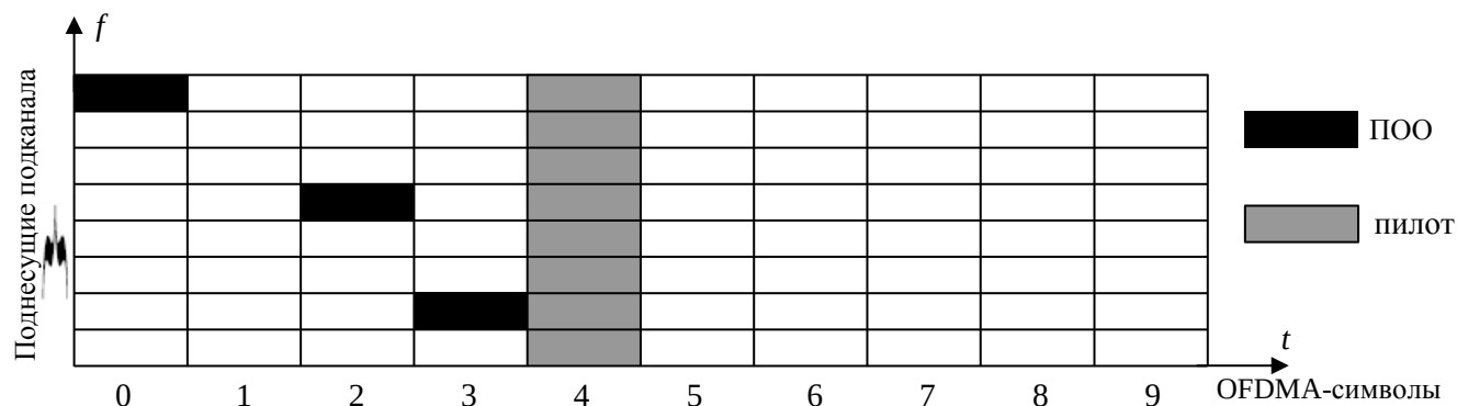
Рисунок 23 – Структура стационарного подканала (ПдК) для супер тайм-слота
