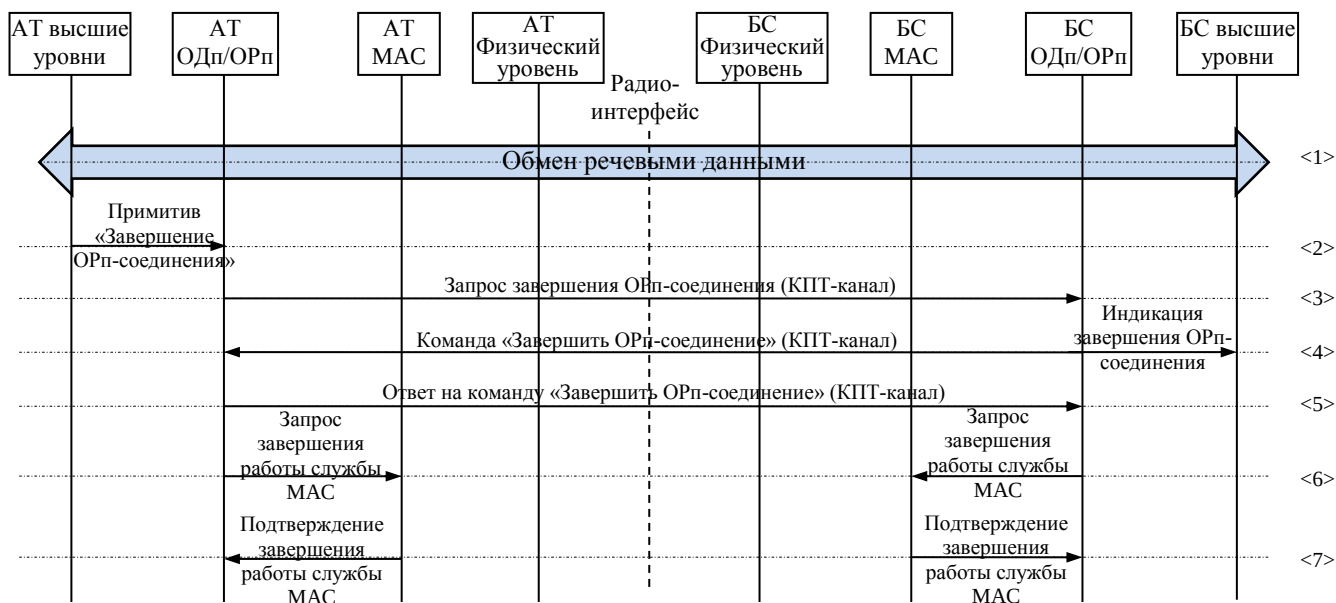
Рисунок 54 – Процедура «Завершение соединения ОРп-подуровня по инициативе АТ»
