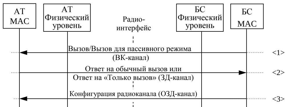
Рисунок 43 –Процедура «Вызов»
