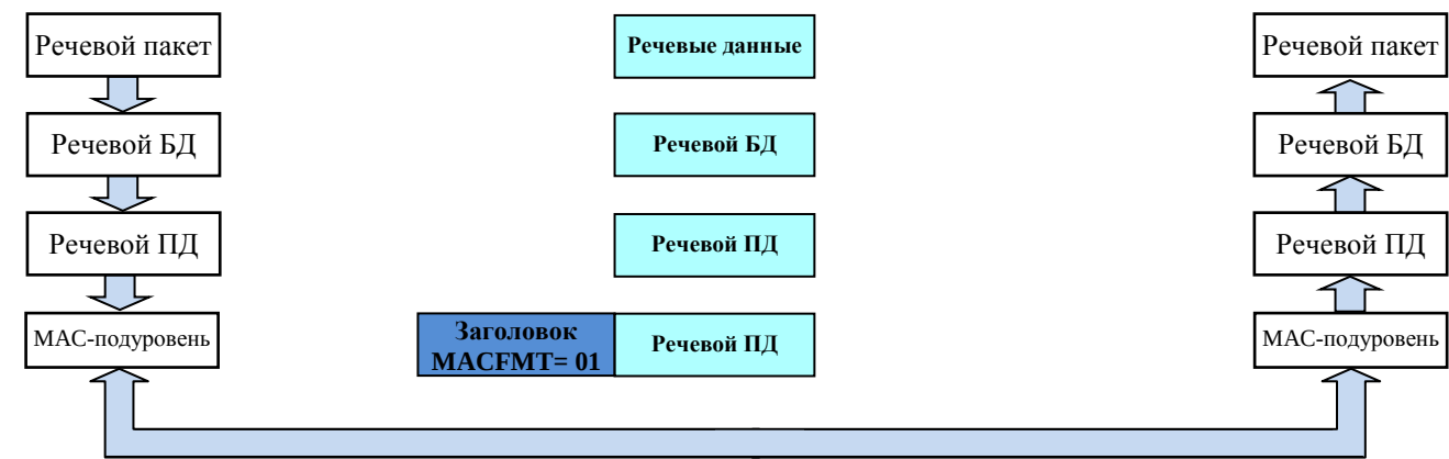
Рисунок 33 – Процесс формирования блоков данных (БД) и пакетов данных (ПД) на ОРп-подуровне
