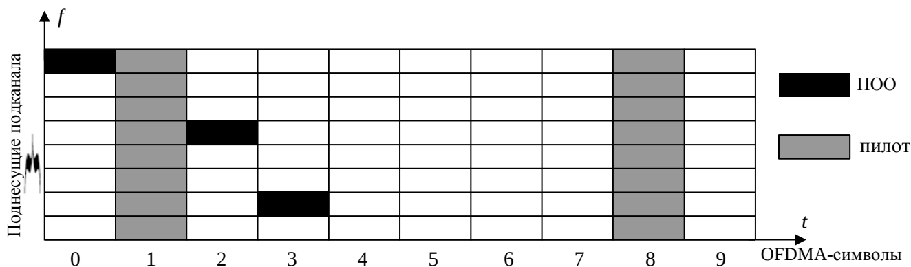
Рисунок 25 – Структура мобильного подканала (ПдК) для супер тайм-слота
