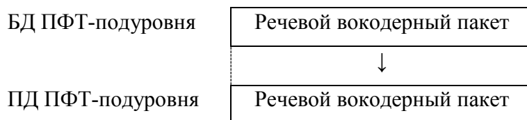
Рисунок 39 – Формирование ПД ПФТ-подуровня из речевого вокодерного пакета
