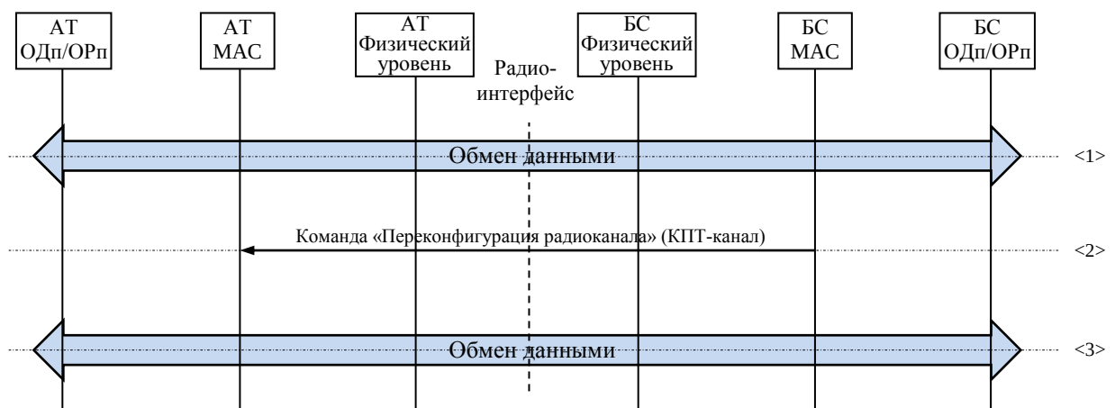
Рисунок 53 – Процедура «Переконфигурация (изменения полосы) радиоканала», осуществляемая БС
