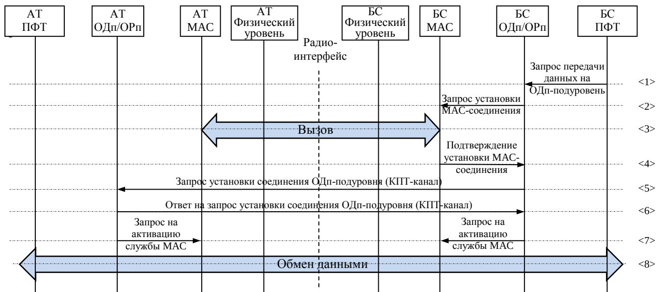
Рисунок 50 –Процедура «Установка соединения ОДп-подуровня по инициативе БС» при отсутствии соединения с MAC-подуровнем АТ
