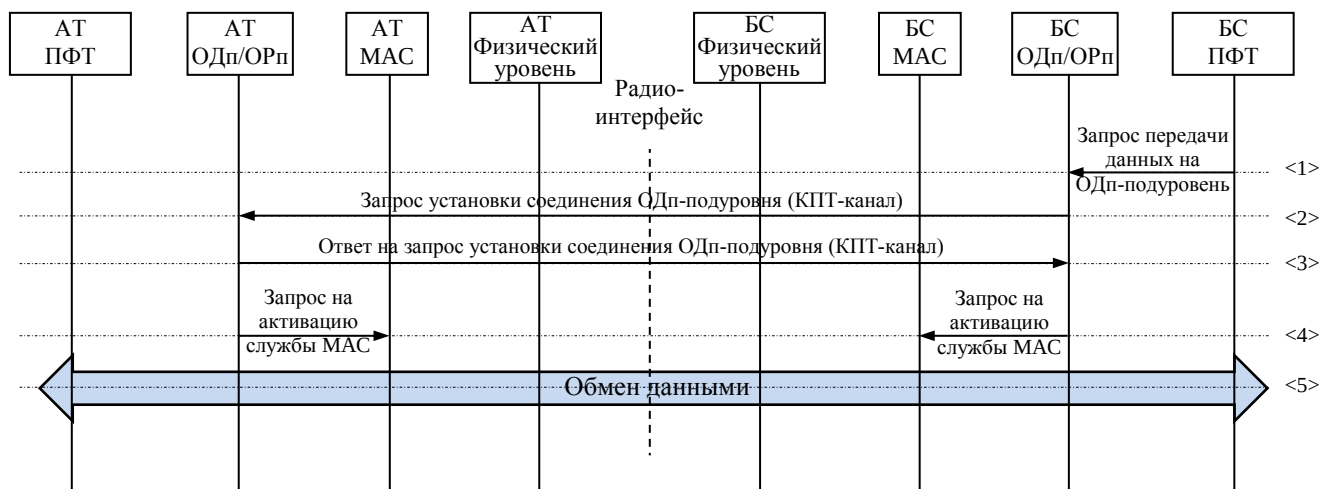
Рисунок 51 –Процедура «Установка соединения ОДп-подуровня по инициативе БС» при наличии соединения с МАС-подуровнем АТ
