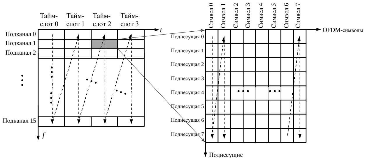
Рисунок 27 – Порядок размещения данных
