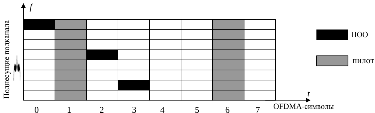
Рисунок 24 – Структура мобильного подканала (ПдК) для обычного тайм-слота
