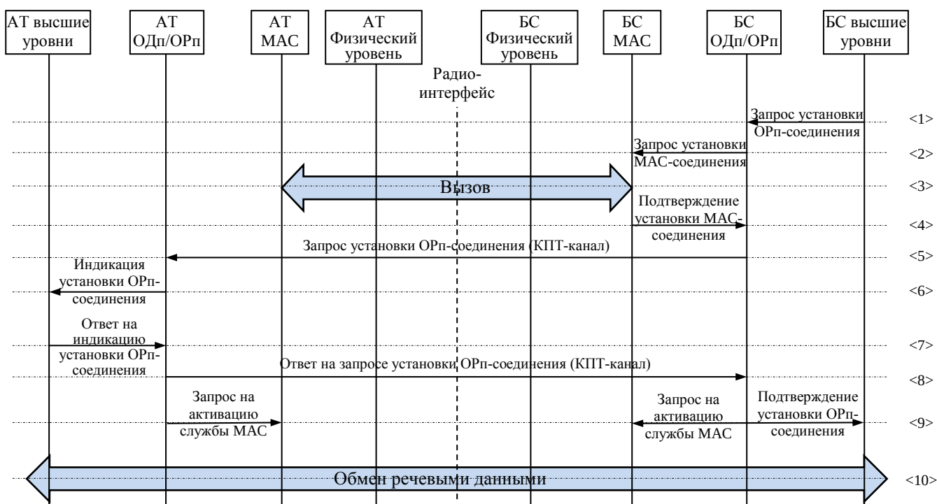
Рисунок 46 –Процедура «Установка соединения ОРп-подуровня по инициативе БС» при отсутствии соединения с МАС-подуровнем АТ
