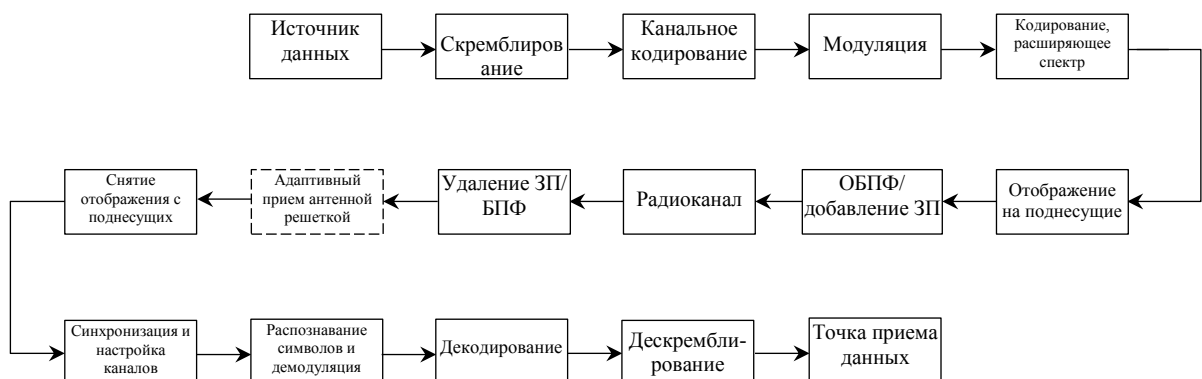
Рисунок 3 – Преобразование потока данных в радиоканале UL
