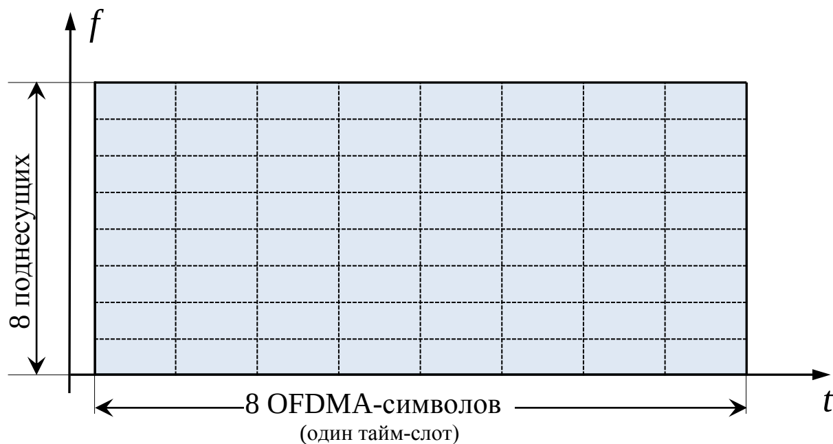
Рисунок 20 – Структура подканала (ПдК) в обычном тайм-слоте
