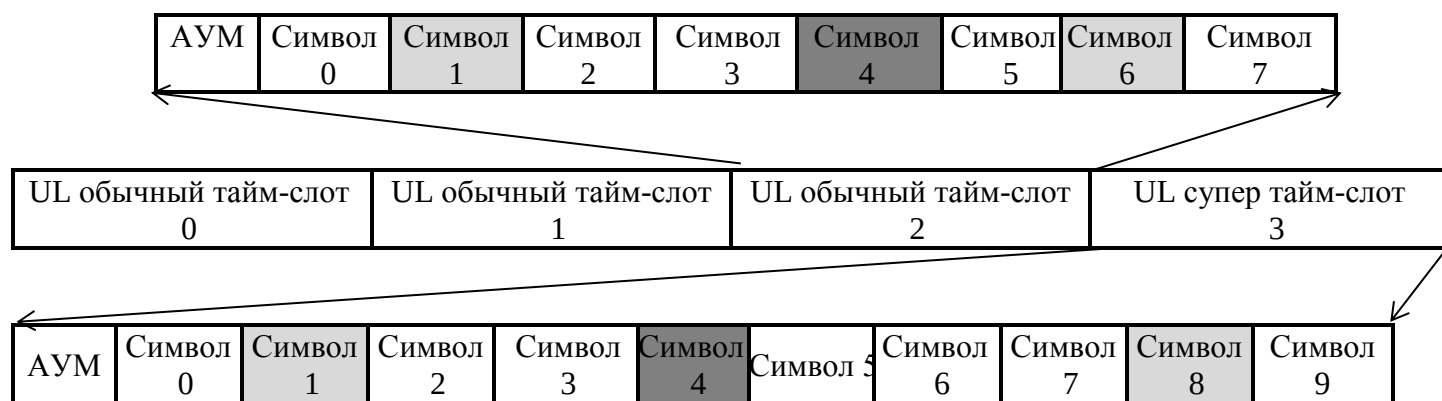
Рисунок 15 – Структура тайм-слотов в кадре трафика в UL длительностью 10 мс
