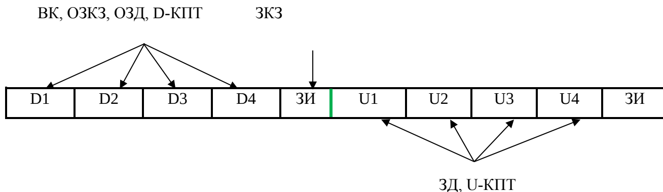
Рисунок 26 – Размещение физических каналов на временных интервалах кадра
