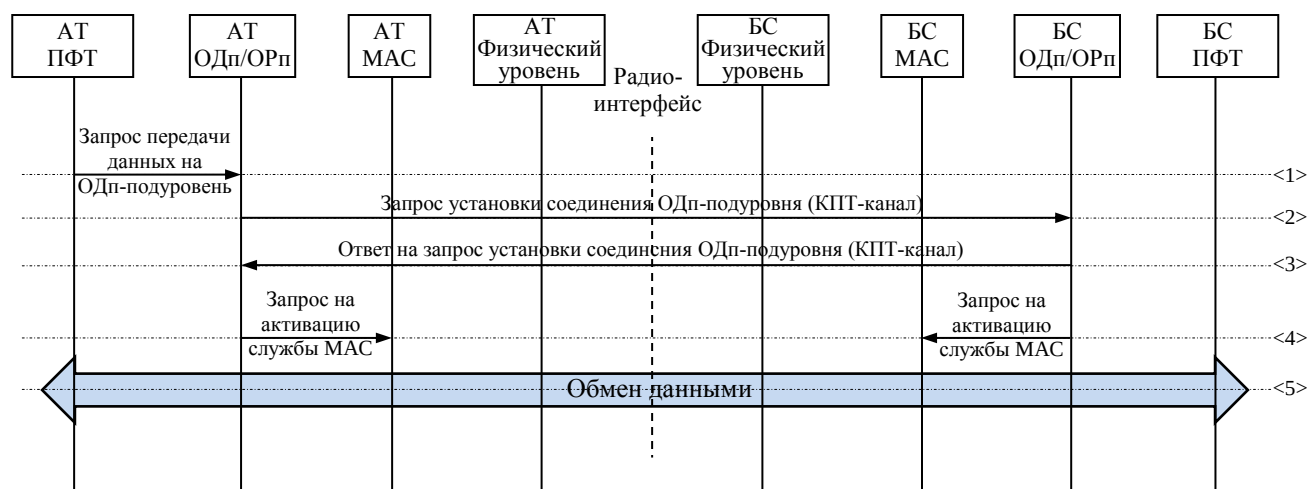
Рисунок 49 –Процедура «Установка соединения ОДп-подуровня по инициативе АТ» при наличии соединения с МАС-подуровнем БС
