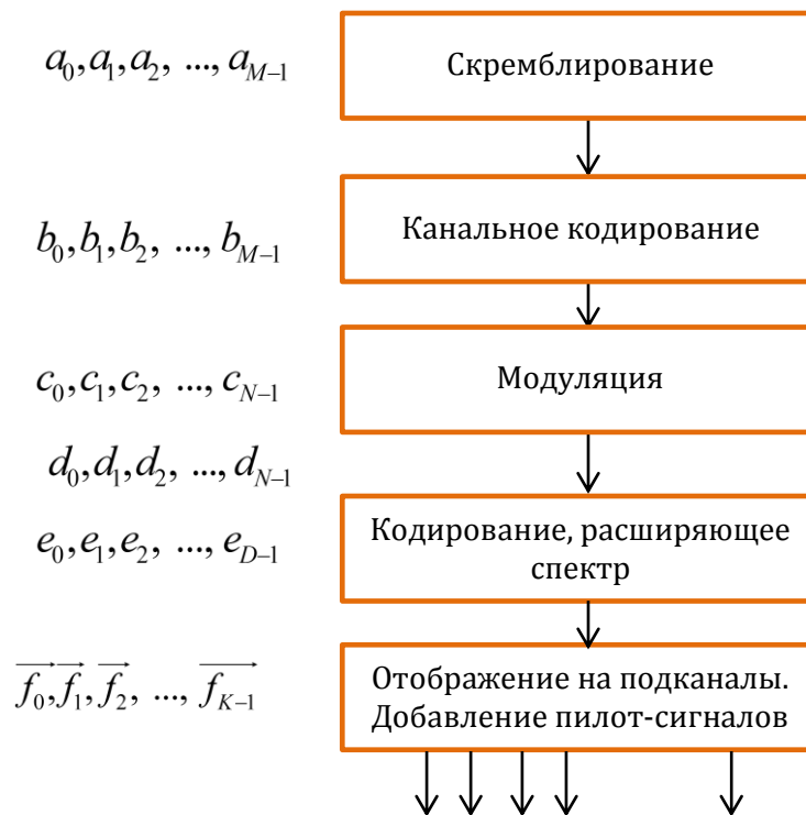
Рисунок 1 – Диаграмма преобразования потока информации на физическом уровне
