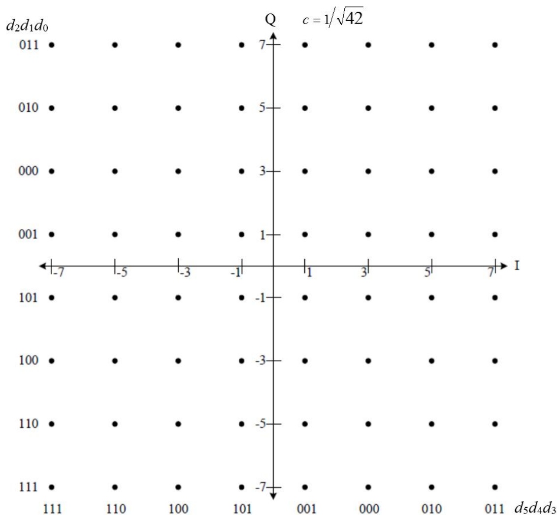
Рисунок 7 – Созвездие 64QAM
