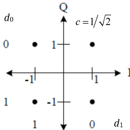
Рисунок 4 – Созвездие QPSK
