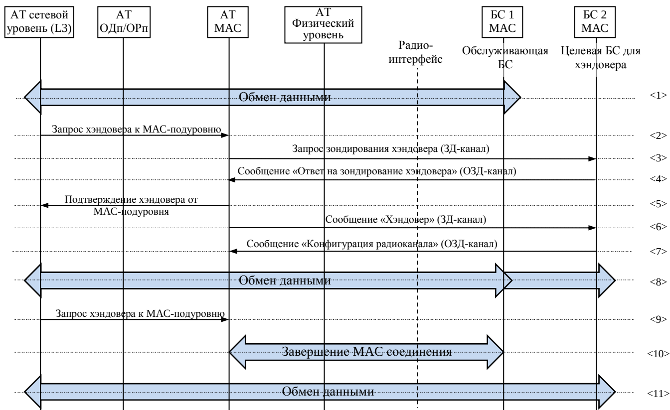
Рисунок 60 – Процедура «Хэндовер»
