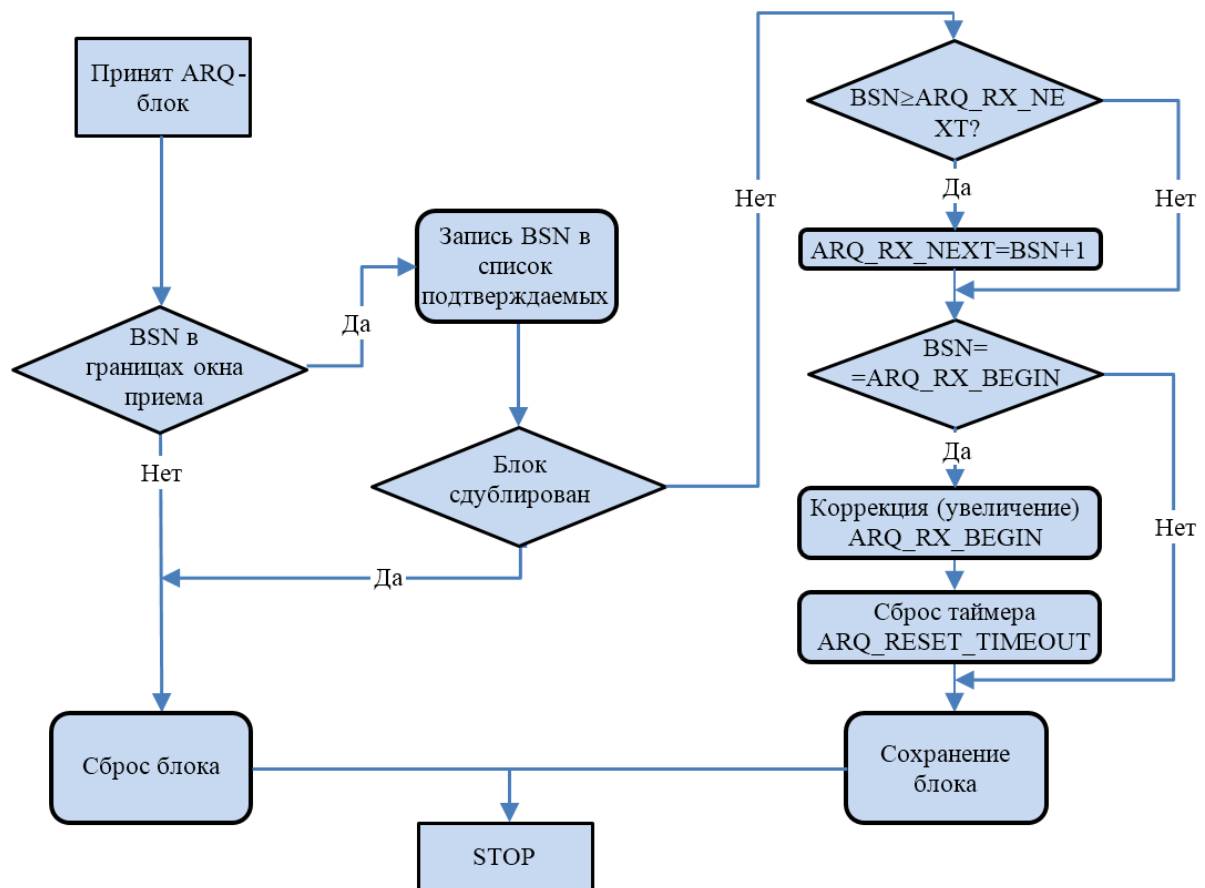
Рисунок 32 – Алгоритм работы в режиме ARQ
