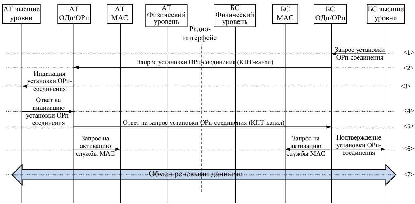
Рисунок 47 – Процедура «Установка соединения ОРп-подуровня по инициативе БС» при наличии соединения с МАС-подуровнем АТ
