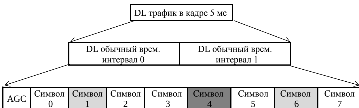
Рисунок 16 – Структура тайм-слотов в кадре трафика в DL длительностью 5 мс
