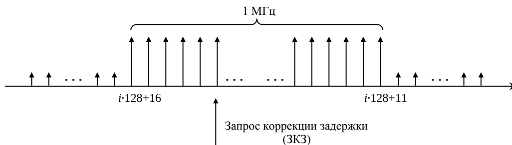
Рисунок 11 – Спектральная структура множества поднесущих, составляющих сигнал ЗКЗ
