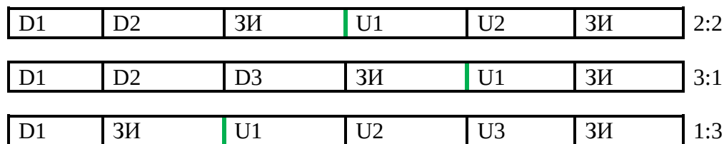
Рисунок 19 – Распределение тайм-слотов в радиолиниях DL/UL для кадра длительностью 5 мс
