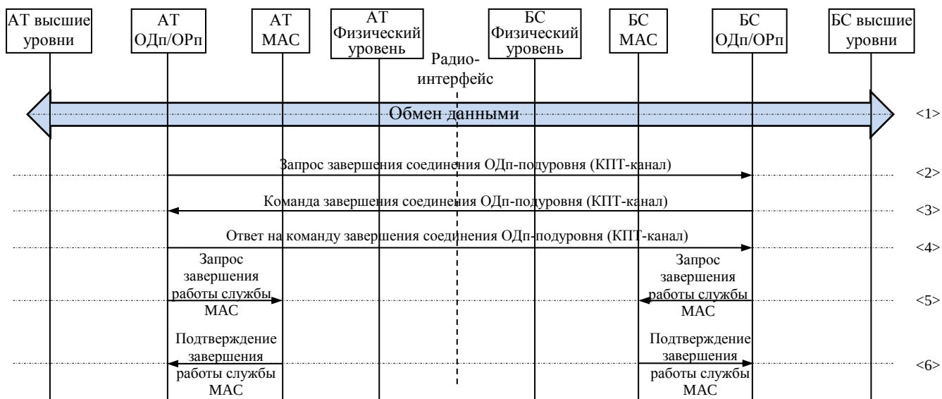
Рисунок 56 – Процедура «Завершение соединения Одп-подуровня по инициативе АТ»
