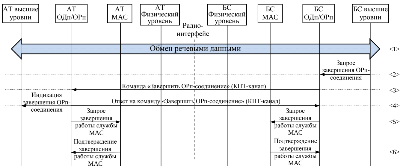
Рисунок 55 – Процедура «Завершение соединения ОРп-подуровня по инициативе БС»
