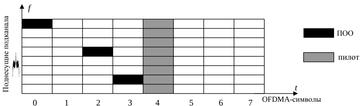
Рисунок 22 – Структура стационарного подканала (ПдК) для обычного тайм-слота
