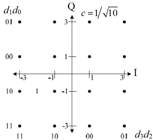
Рисунок 6 – Созвездие 16QAM
