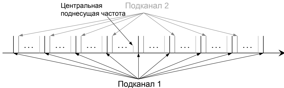
Рисунок 9 – Частотно-спектральная структура OFDMA-символа
