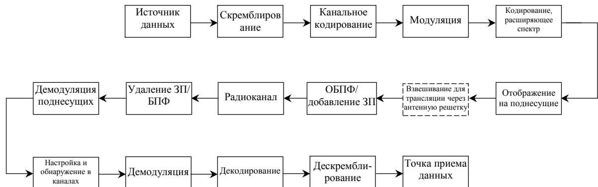
Рисунок 2 – Преобразование потока данных в радиоканале DL
