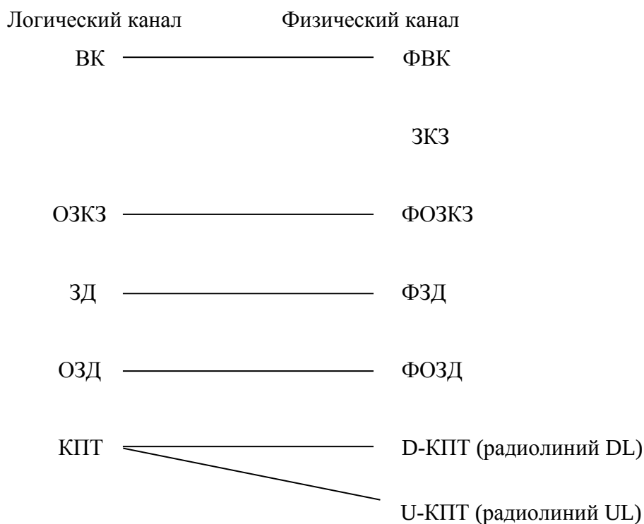
Рисунок 29 – Отображение логических каналов на физические каналы
